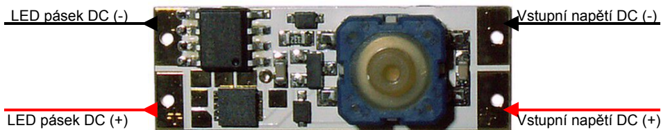
Obr. 1 - Zapojení vývodů modulu stmívače
